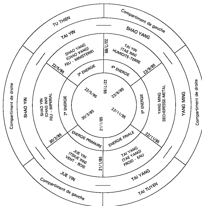
Cette figure indique le Tai Yin dans le compartiment central de Tu Thiên et le Tai Yang dans le compartiment central de Tai Tuyen. Les deux cercles intérieurs indiquent les six « pas » de l'énergie hôtesse, invariables pendant toutes les années. Les deux cercles extérieurs indiquent les six « pas » de l'énergie invitée, l'emplacement de Tu Thiên et de Tai Tuyen et de leurs compartiments pour l'année : Yi-Chou (I-Tchréou : 2-II) ou Métal-Buffle.
